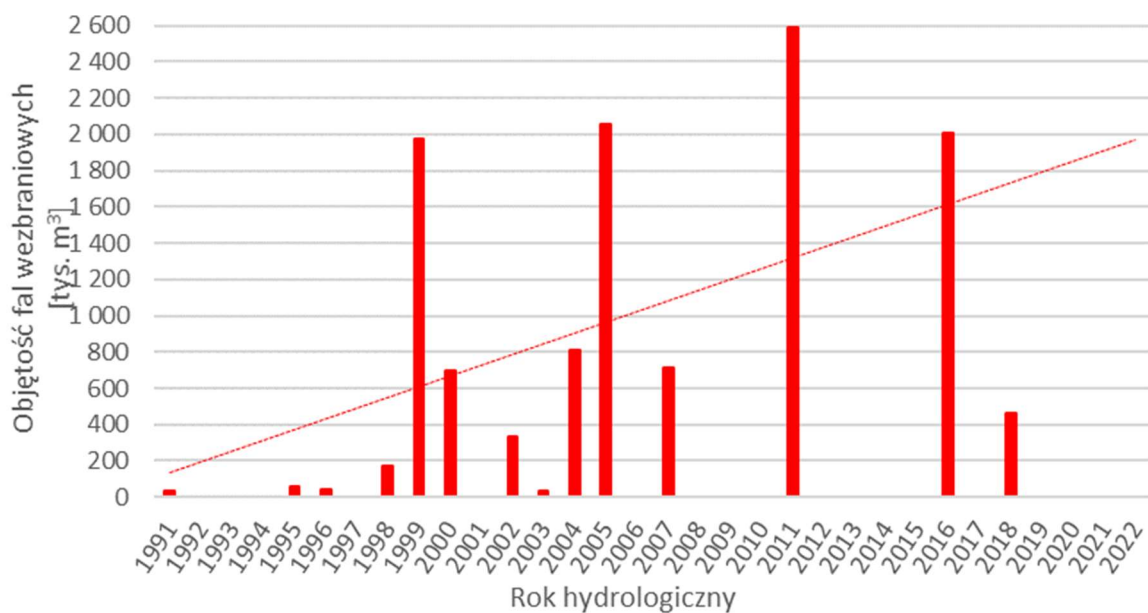
Rys.96. Objętość fal wezbraniowych w latach hydrologicznych (rz. Reda, profil Wejherowo)
