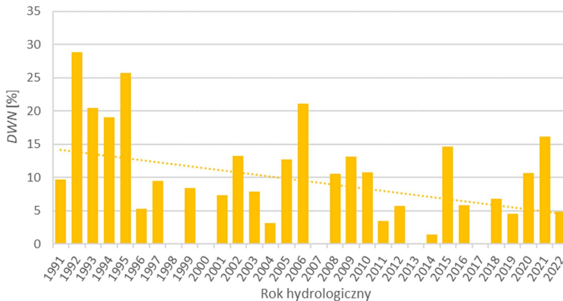
Rys.95. Deficyt względnego odpływu niżówkowego w poszczególnych latach hydrologicznych (profil Wejherowo, rz. Reda)
