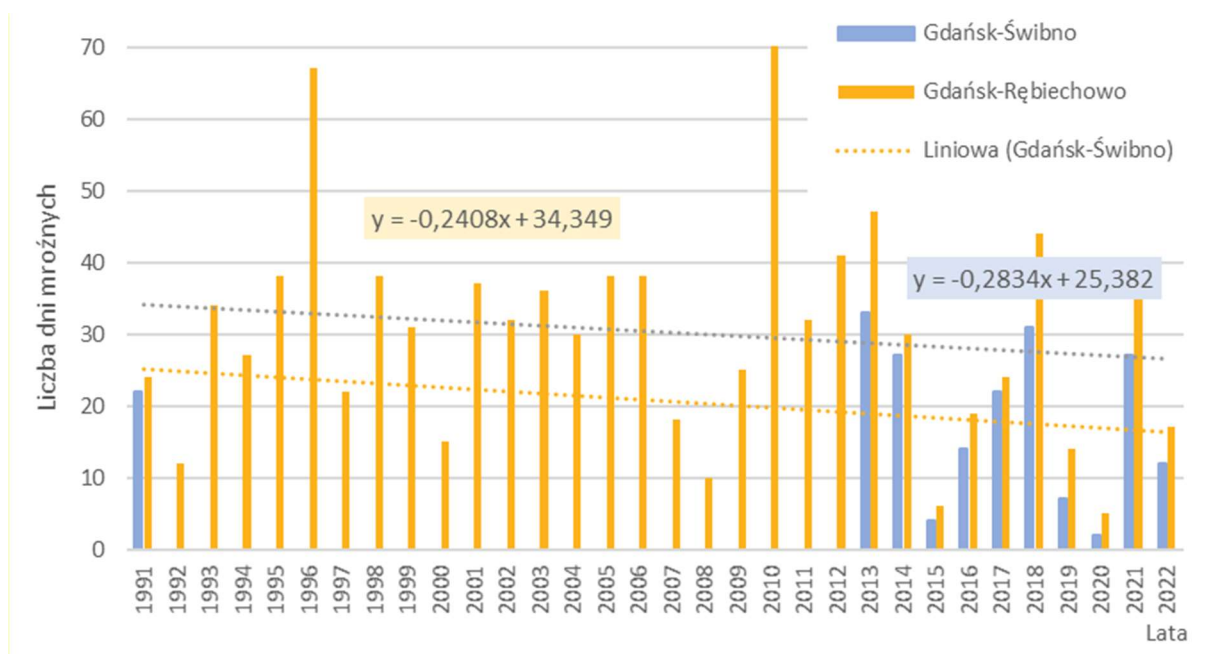
Rys.13. Liczba dni mroźnych (T max <0°C), Gdańsk-Rębiechowo i Gdańsk-Świbno
